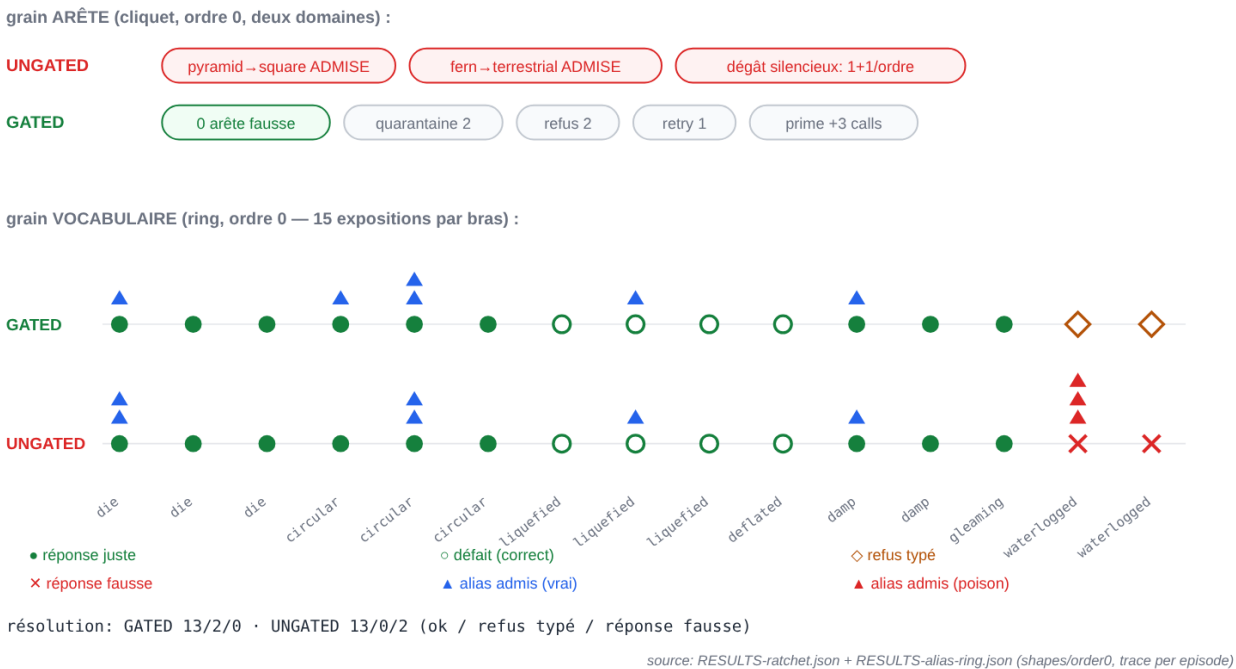
Figure F6 — le cliquet, généré des traces réelles (ordre 0) : en haut le grain arête (UNGATED absorbe pyramid→square et fern→terrestrial, dégât silencieux ; GATED zéro arête fausse à prime bornée) ; en bas la timeline du ring (§6.6), exposition par exposition — les admissions vraies (▲ bleu), le poison absorbé par UNGATED seul (▲ rouge, épisodes « détrempés » (waterlogged)), les réponses fausses (×) converties en refus typés (◇) côté GATED, à résolution égale 13 == 13.
