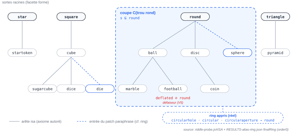
Figure F2 — le treillis isa déclaré du domaine formes (lu dans la source du probe), la restriction du trou rond dessinée comme coupe, le défaiseur deflated ∅ round (V5), et le ring de synonymes réellement appris dans le run du ring ( circularhole · circular · circularaperture → round ), attaché à la clé de la sorte.
